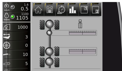
Anzeige Durchrodefahrt aktiv siehe Seite 201
