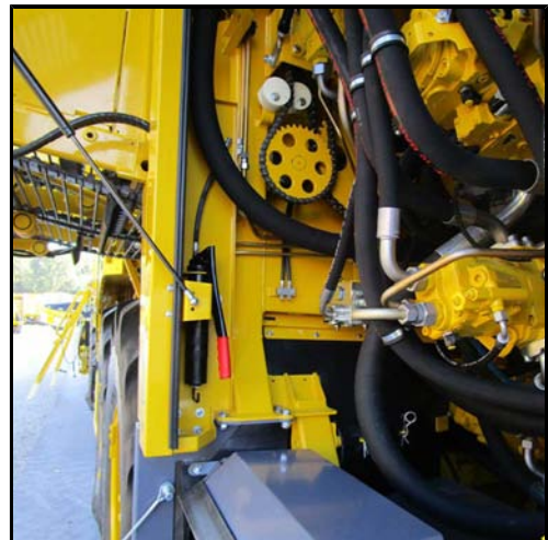
Halterung für Fettpresse
