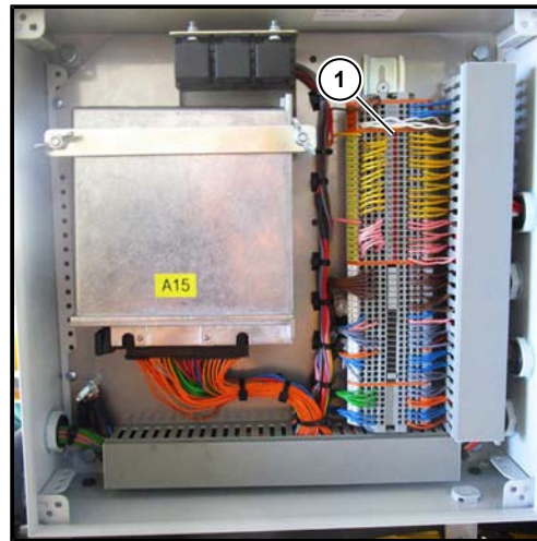
(1) LED elektronische Sicherung im Roderelektrikkasten
