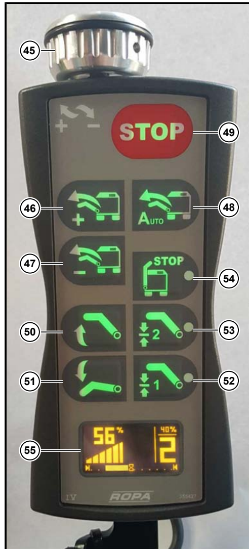
Tastenübersicht siehe Seite 88
