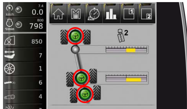
Hinterräder werden von Autopilot gelenkt
