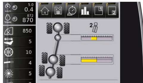
Anzeige Schongang links aktiv
