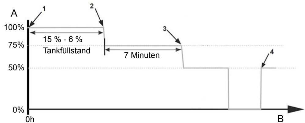
A Motordrehmoment B Zeitachse
