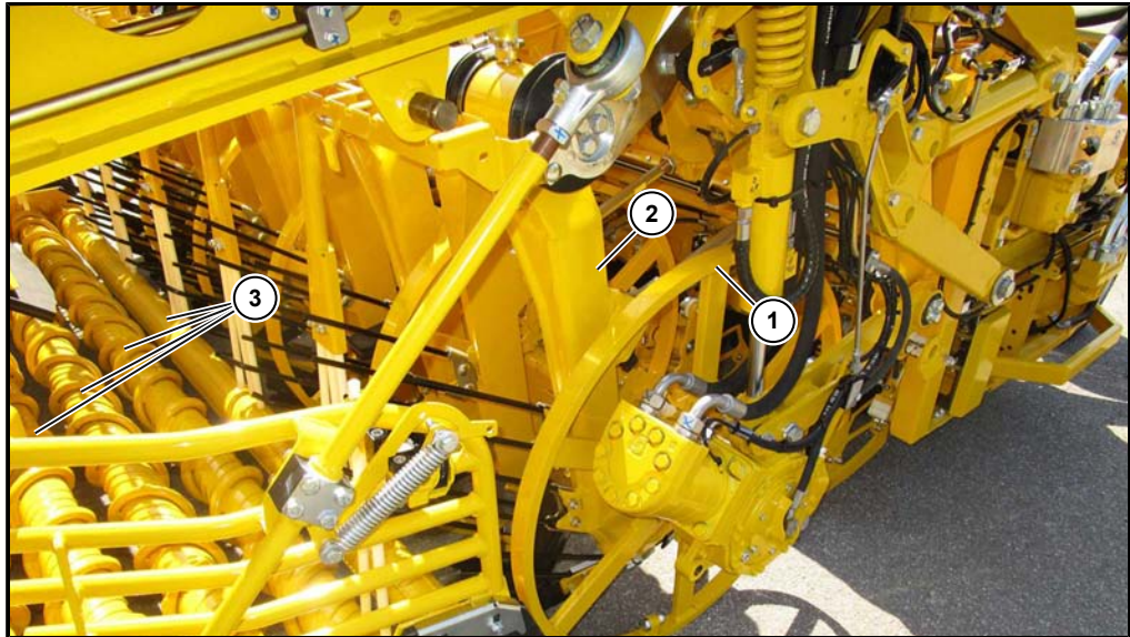
Rodeaggregat, zur besseren Übersicht ohne Schutzvorrichtung abgebildet
