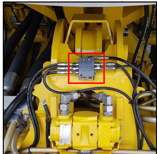
Hauptverteiler Roder und Schlegler
