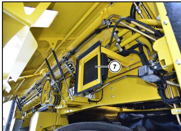
(7) Ölkühler Vorsatzgetriebe
