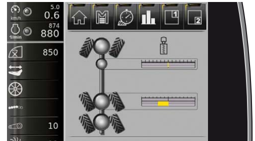
Anzeige bei Starrfahrt siehe Seite 205
