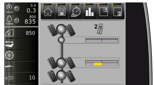
Anzeige Hundegang aktiv siehe Seite 206
