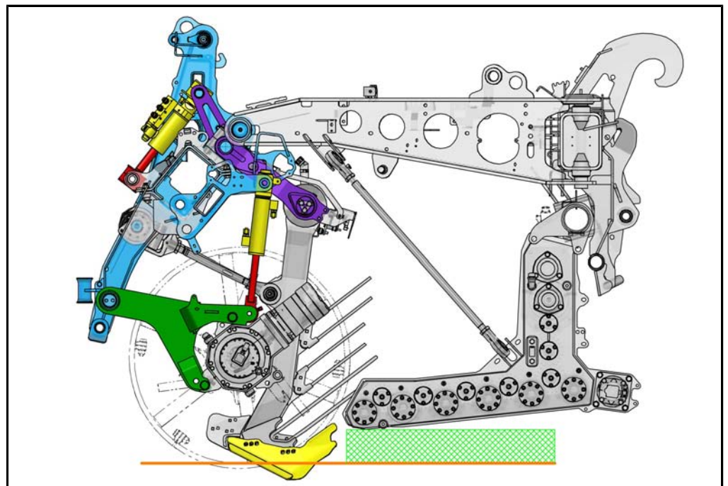
Walzengang hoch
