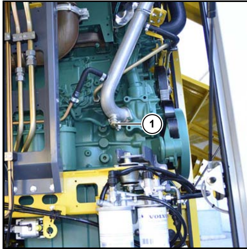
(1) Ablassventil für Kühlflüssigkeit am Kühlwasserrohr
