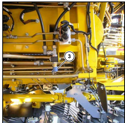
(3) Druckluftkupplung neben Siebsterkamera
