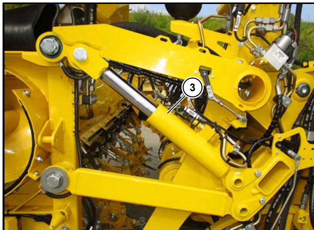
(3) Schleglerentlastungszyylinder
