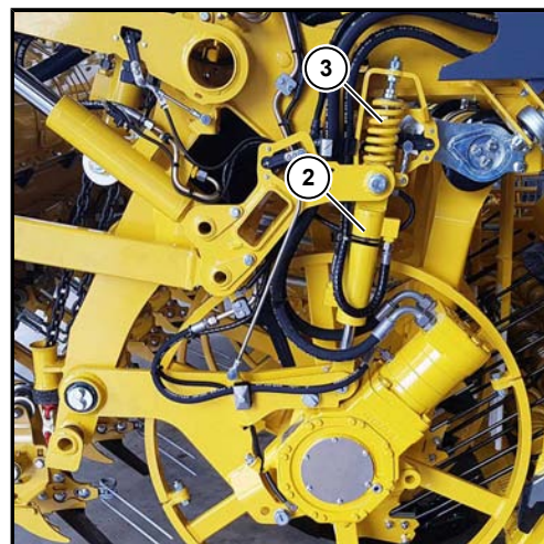
(2) Zylinder-Walzenganghöhenverstellung
