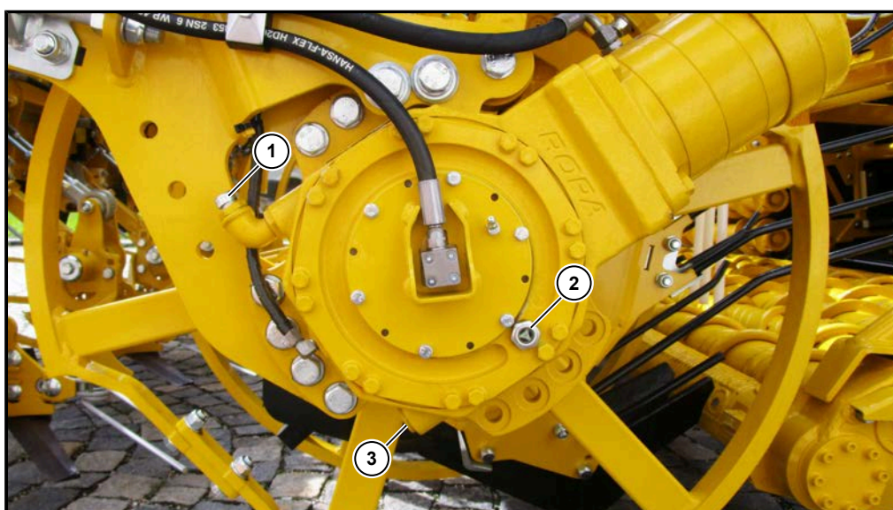
Bild zeigt Ausführung ab 2018
