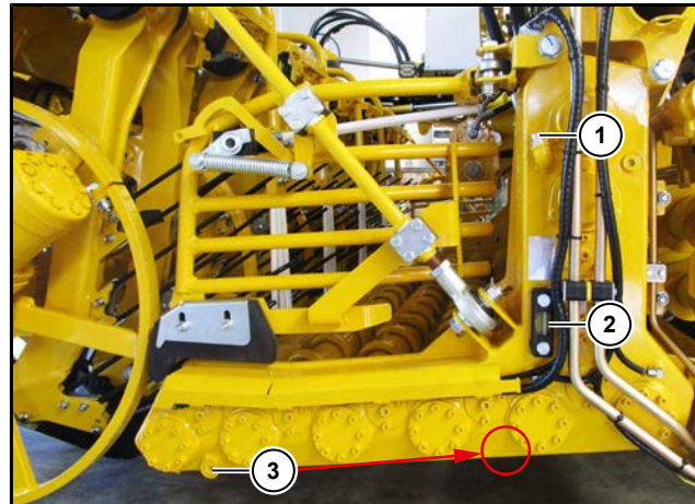
Bild zeigt Ausführung 2017
