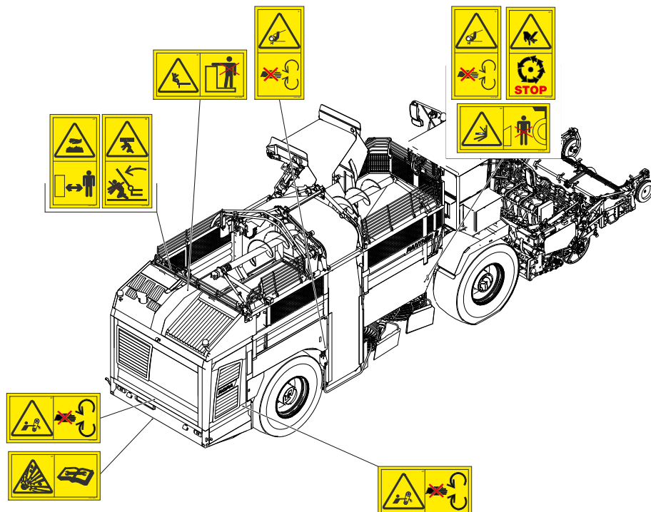
Abbildung zeigt beispielhaft eine Maschine mit Erntevorsatz RR-45 und RIS-45
