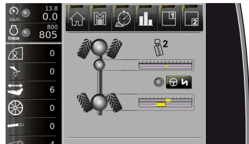
Anzeige bei Starrfahrt siehe Seite 208
