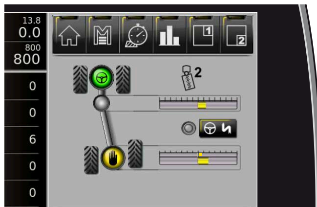
Hinterräder werden von Joystick gelenkt
