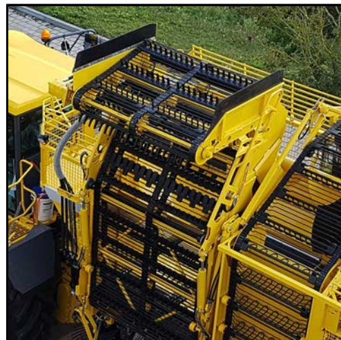
Entladebandknickteil 1 und 2 in Rodestellung
