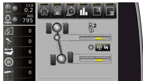
Anzeige Schongang rechts aktiv
