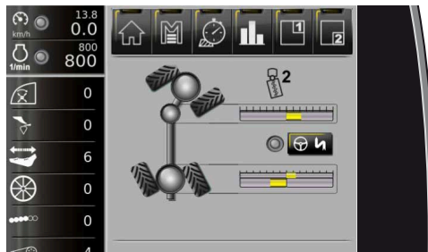
Anzeige bei aktiver Wendefahrt siehe Seite 208
