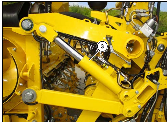
(3) Schleglerentlastungszylinder
