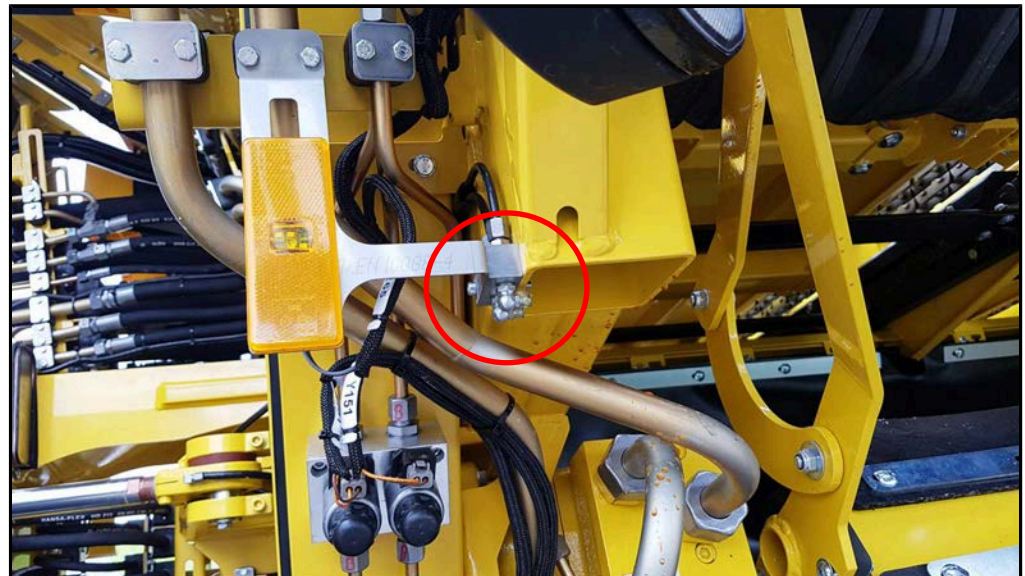
Schmiernippelblock am Getriebe Querkratzboden
