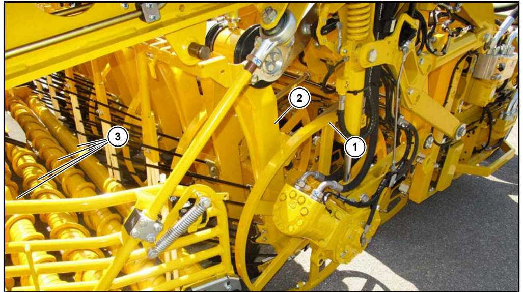
Rodeaggregat, zur besseren Übersicht ohne Schutzvorrichtung abgebildet
