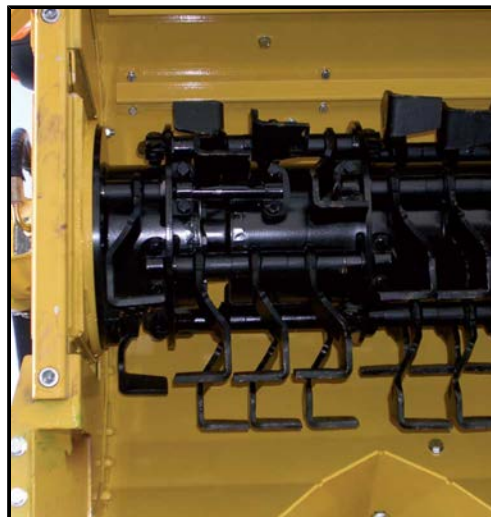
Schleglermesser und Klemmlaschen beim RIS
