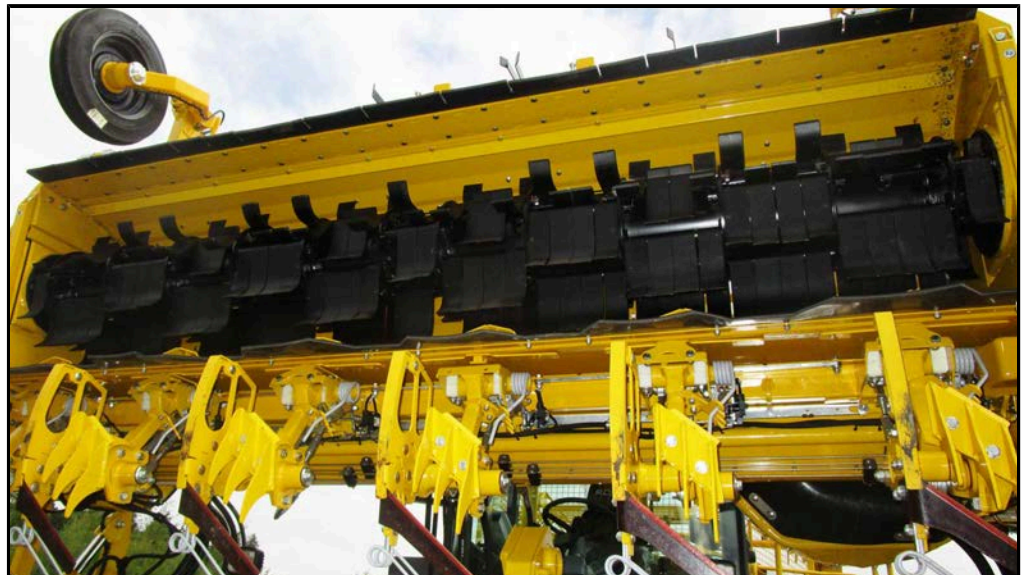
RAS-Schlegler von unten
