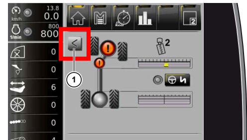
Anzeige bei erforderlicher Synchronisierung siehe Seite 200
