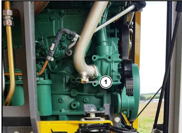
(1) Ablassventil für Kühflüssigkeit am Kühlwasserrohr
