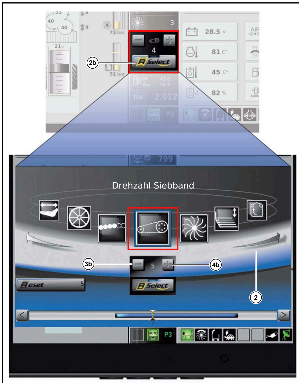
R-Select Modus (Beispielhaft Drehzahl Siebband ausgewählt)
