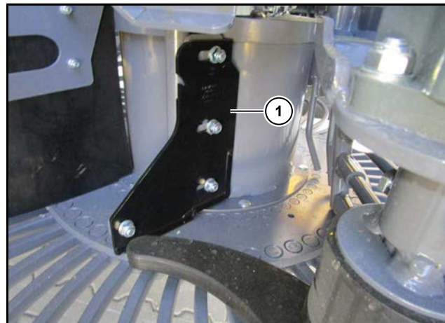
(1) Siebsterne Abstreifer
