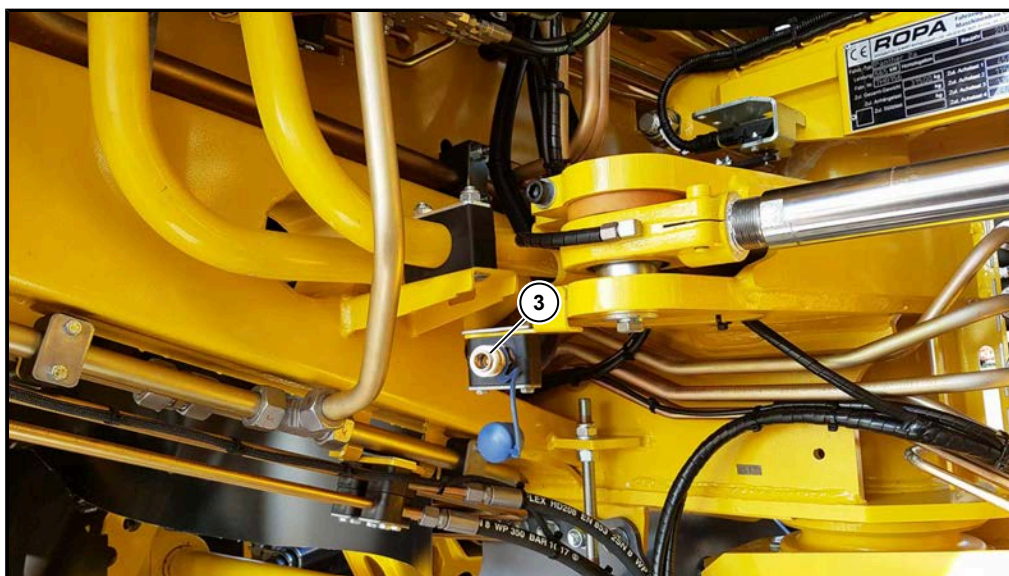
(3) Druckluftkupplung vorne rechts am Knick
