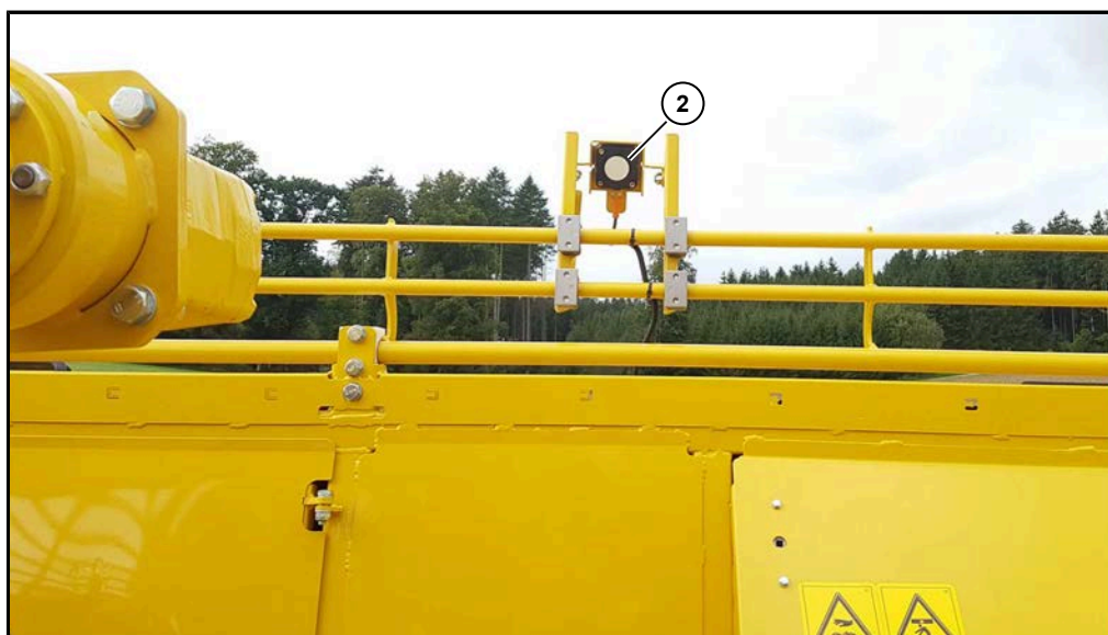
(2) Ultraschallsensor hinten
