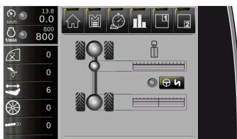
Anzeige Durchrodefahrt aktiv siehe Seite 204
