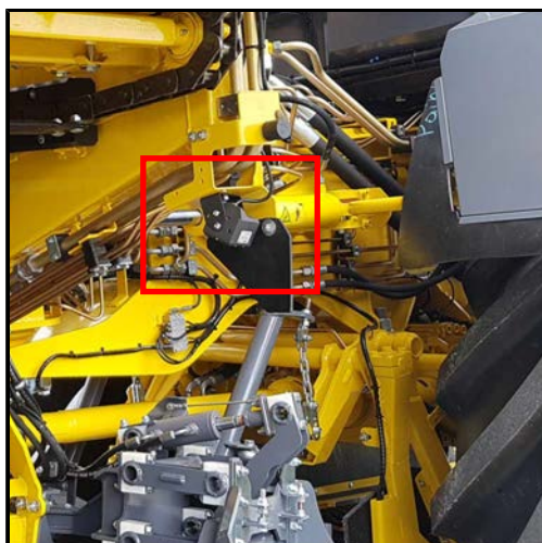
Siebsterne-Kamera
