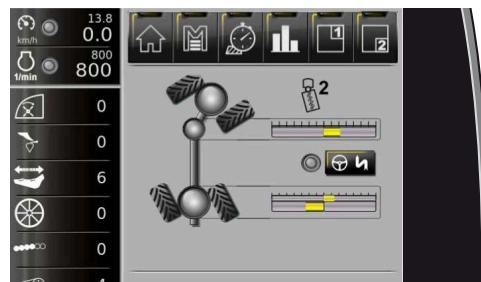
Anzeige bei aktiver Wendefahrt siehe Seite 201
