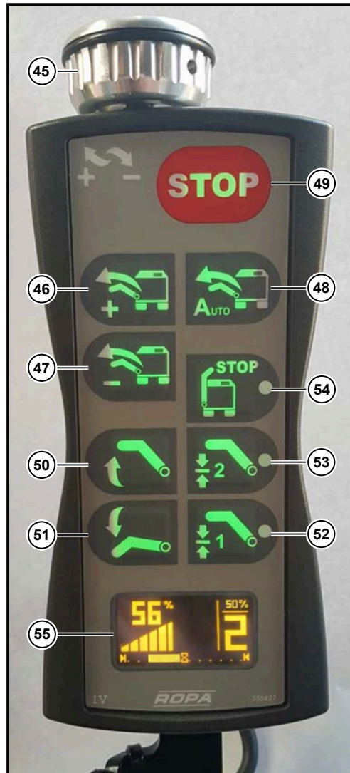
Tastenübersicht siehe Seite 90
